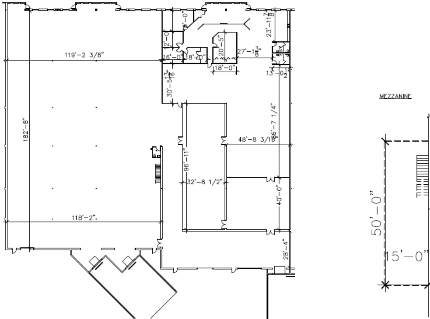
TENANT "E-G" FLOOR PLAN 43,077 S.F.
